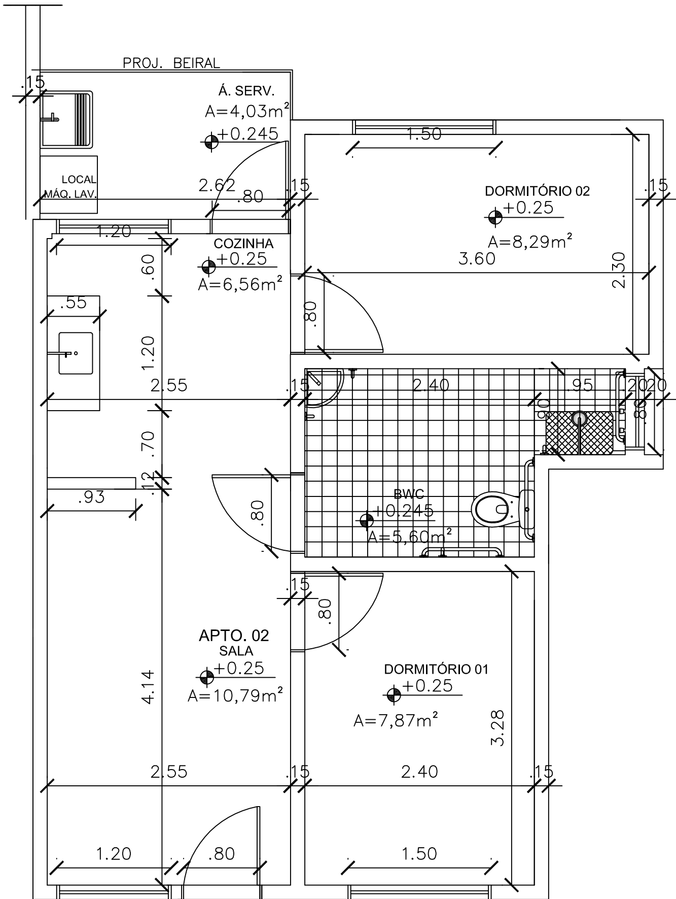
PLANTA BAIXA - APARTAMENTO ACESSÍVEL
