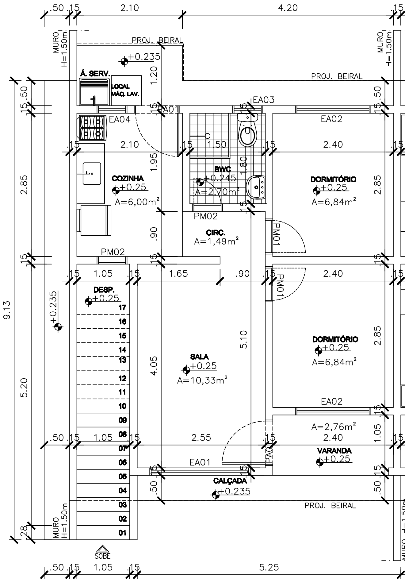
PLANTA BAIXA - PAVTO. TÉRREO - 48,33m 2
