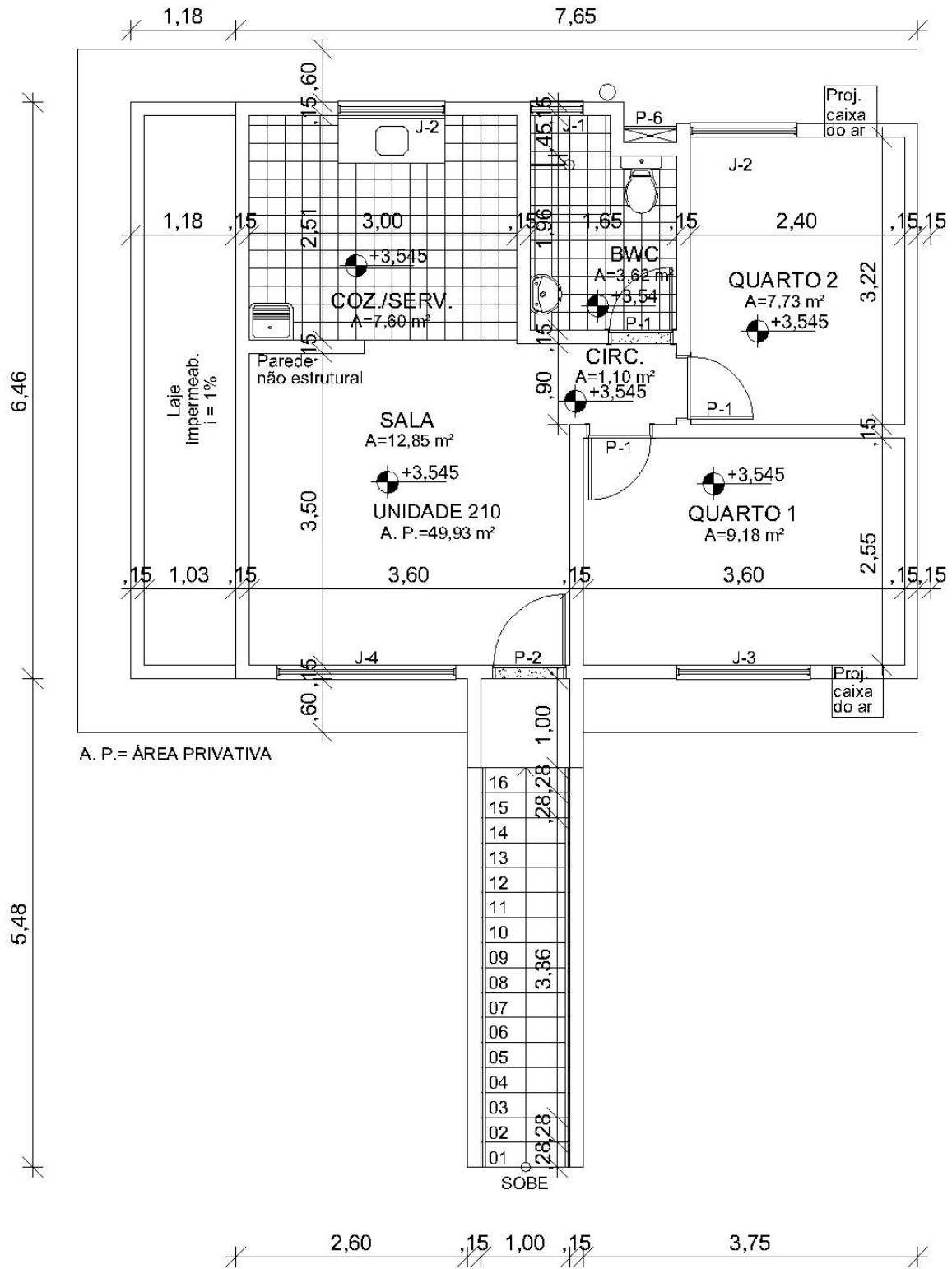
PLANTA BAIXA - PAVTO. SUPERIOR - 49,93m 2
