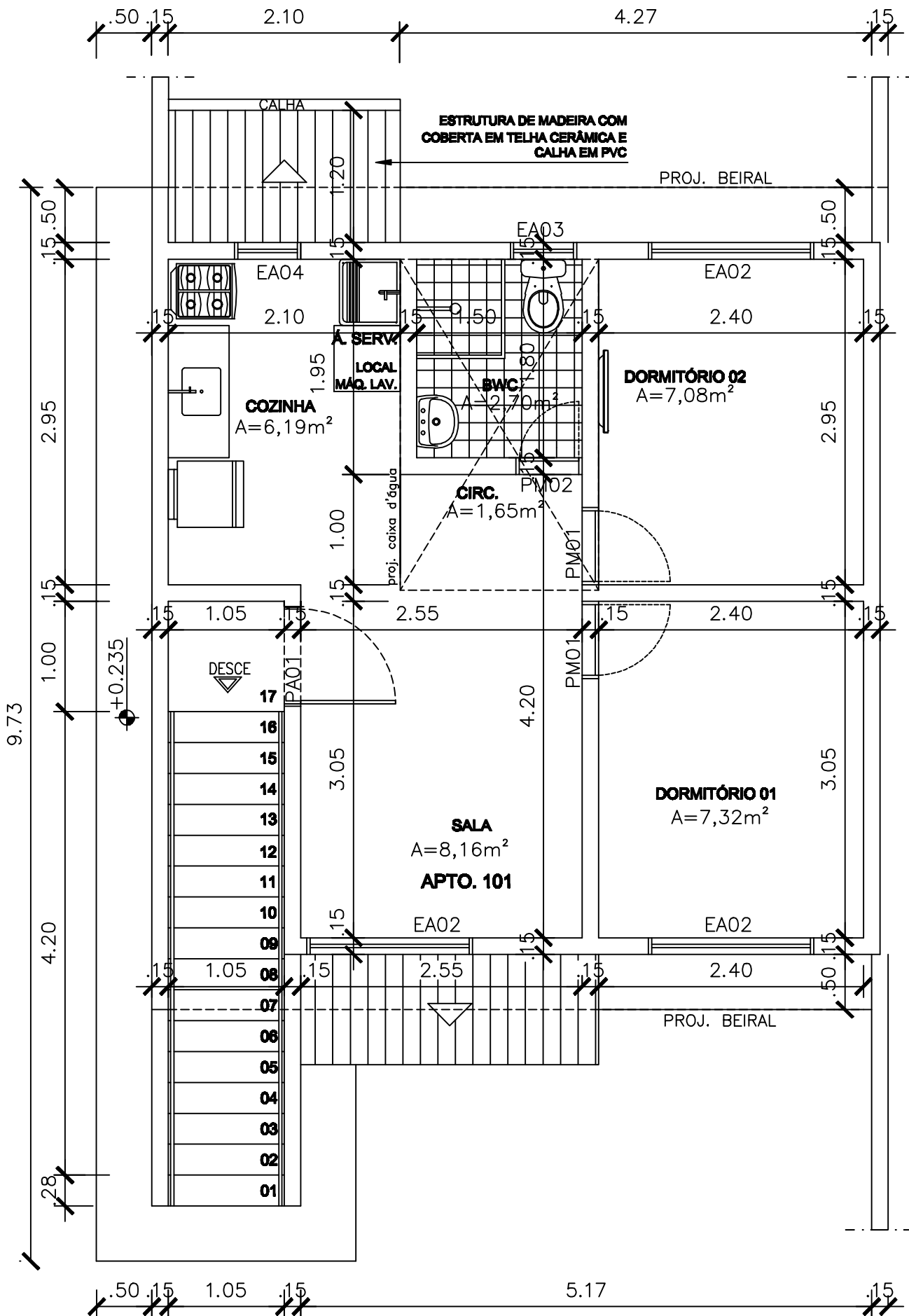
PLANTA BAIXA – PAVTO. SUPERIOR – 43,16m^2
