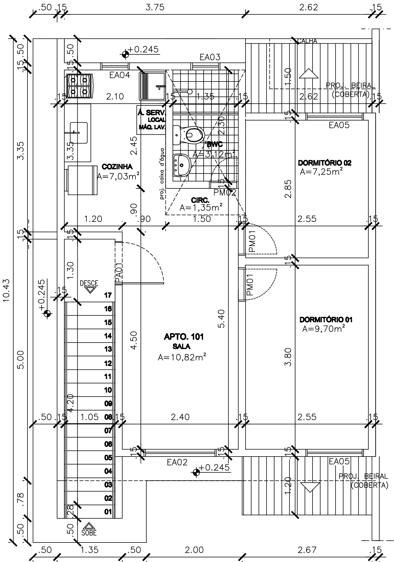
PLANTA BAIXA – PAVTO. SUPERIOR – 51,59m^2
