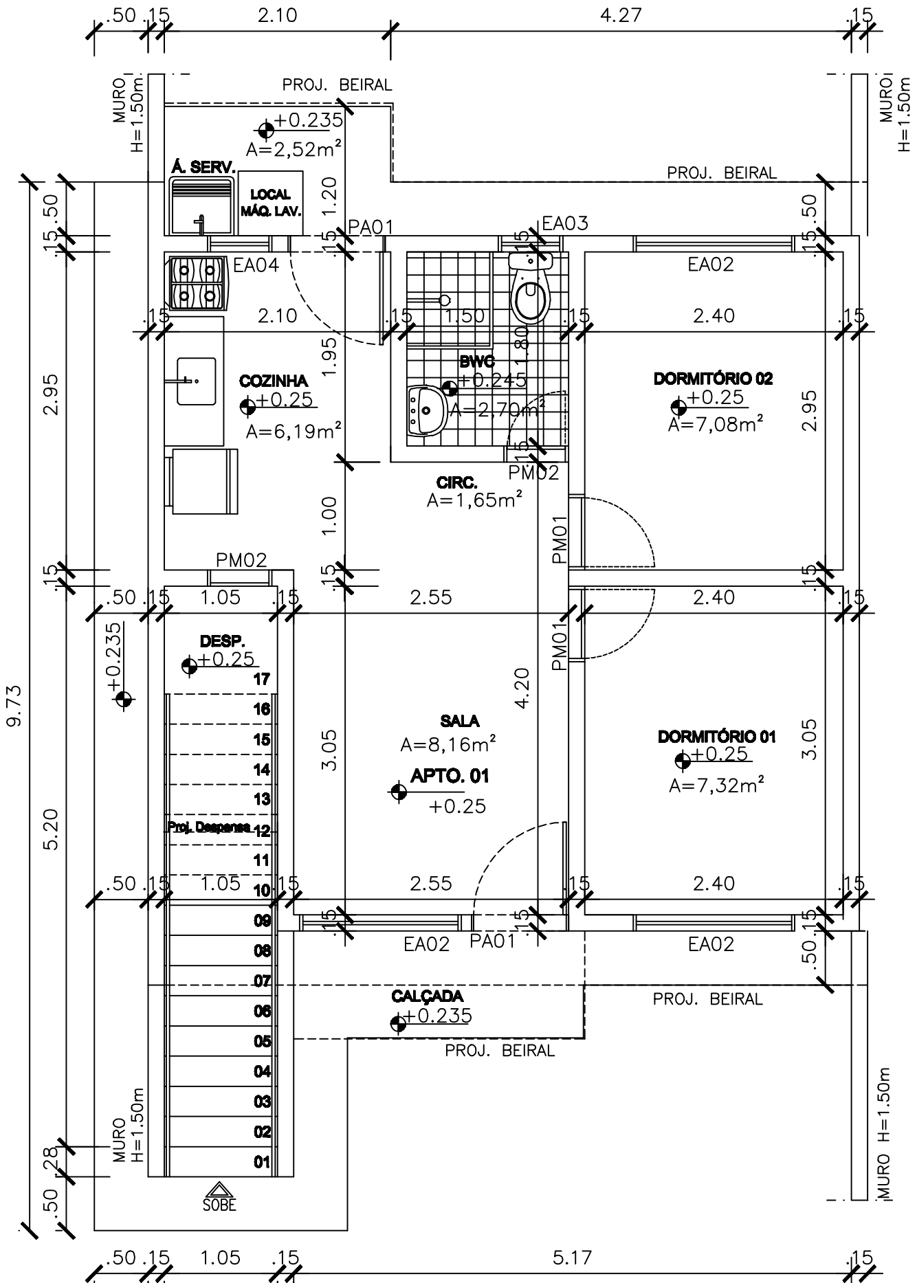
PLANTA BAIXA – PAVTO. TÉRREO – 44,06m 2
