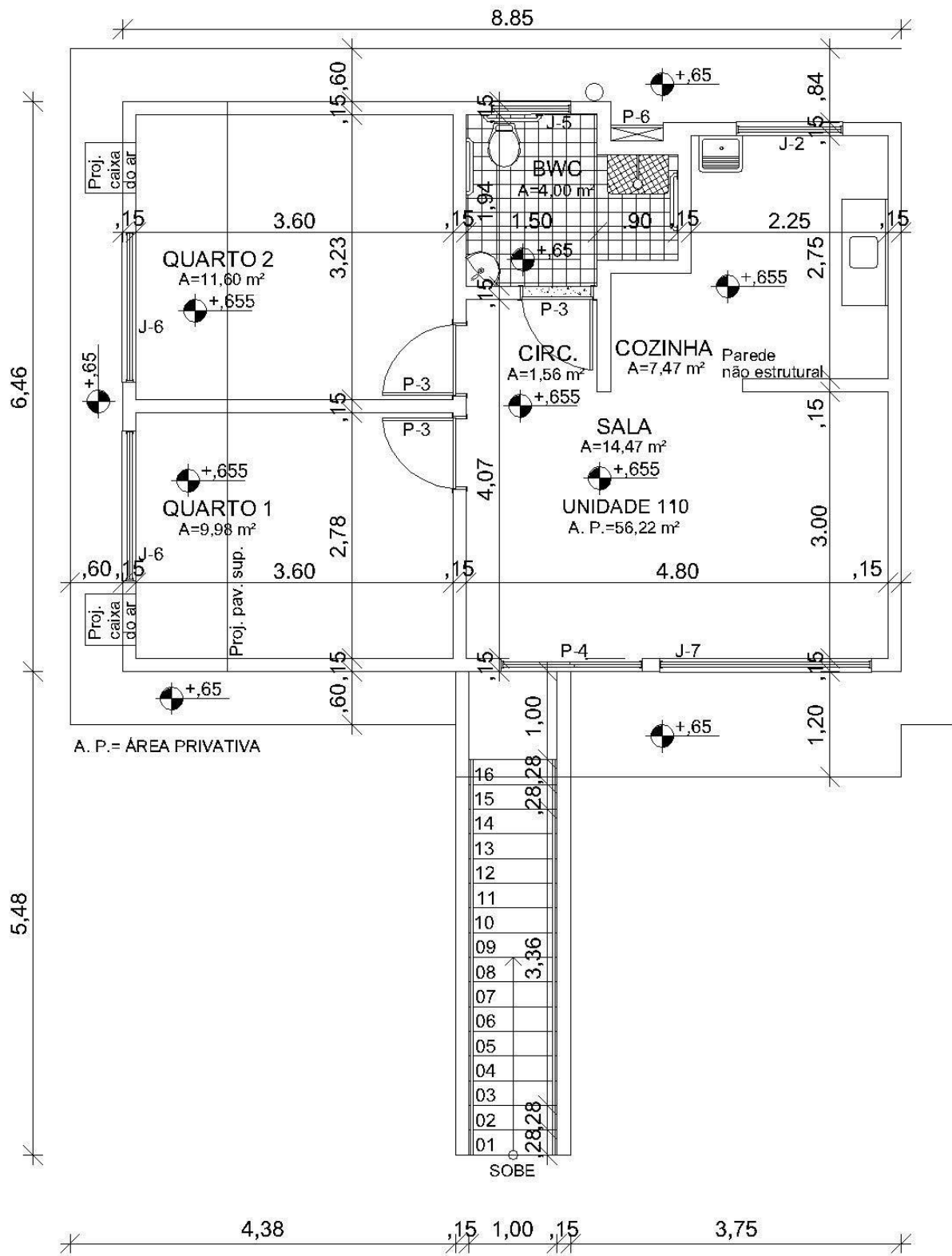
PLANTA BAIXA - PAVTO. TÉRREO - UNIDADE ACESSÍVEL - 56,22m 2
