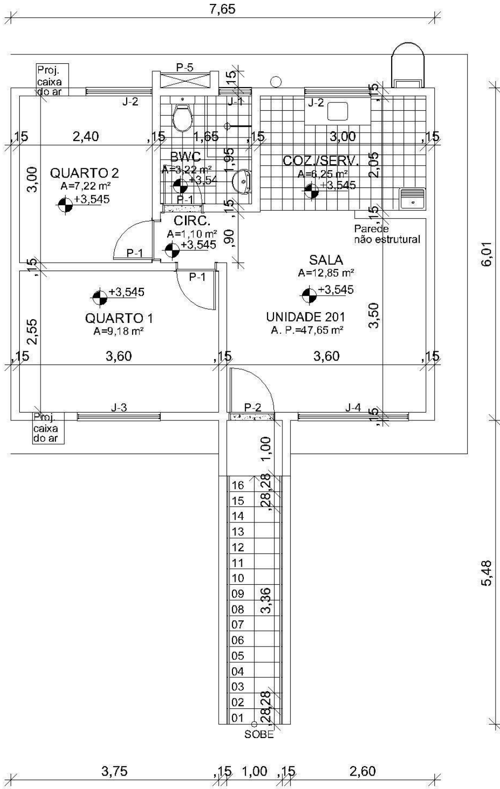
PLANTA BAIXA - PAVTO. SUPERIOR - 47,65m 2
